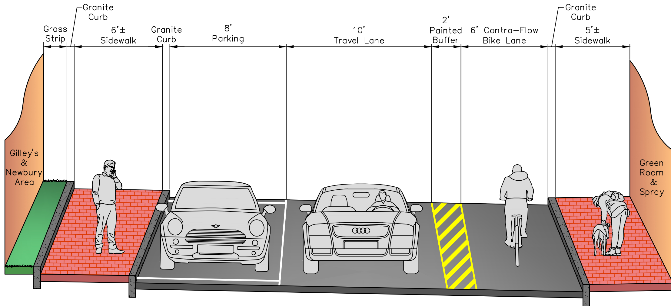
MID BLOCK (STA. 3+50) SCALE: 1" = 4'
